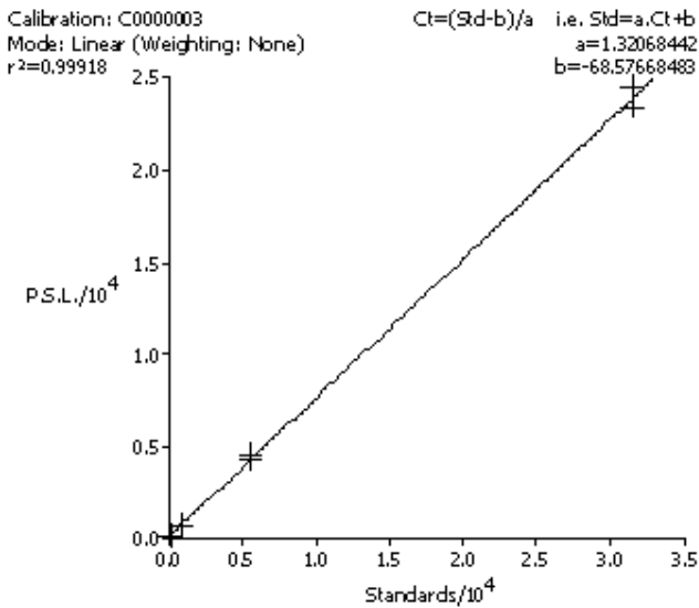
QWBAの解析例（検量線）
